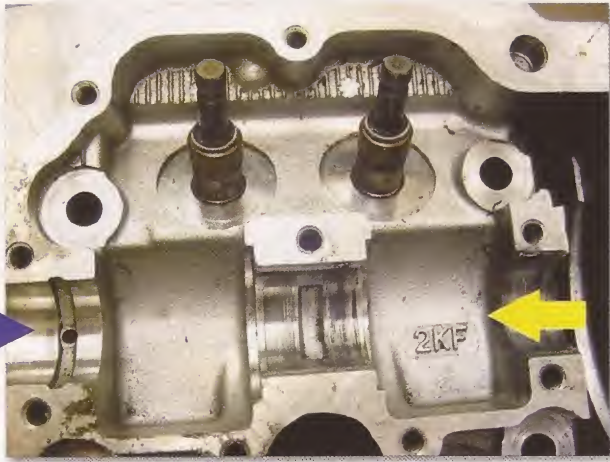
Soporte de árbol de levas
